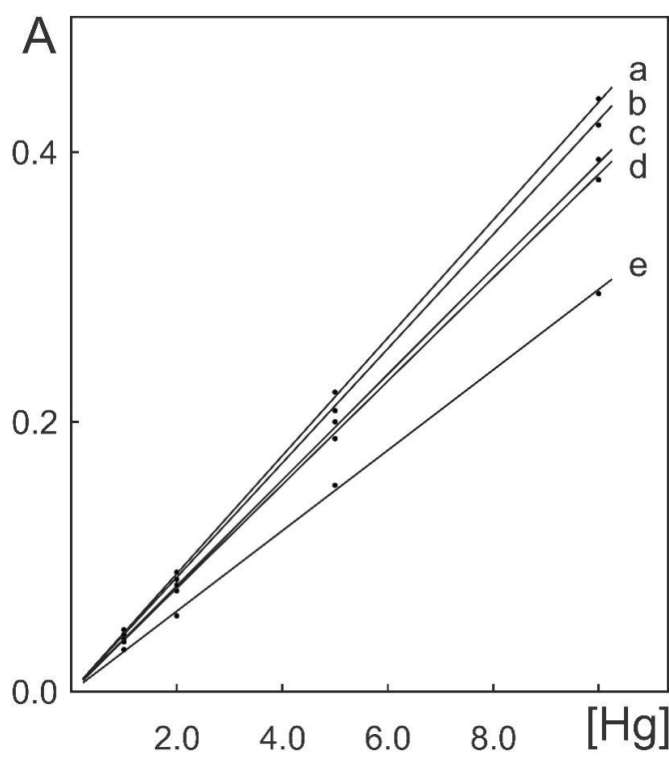
Figura 2 - Influência do fluxo de argônio nas curvas analíticas; a, b, c, d, e: Fluxos de Ar de 3,6; 3,0; 2,5; 4,5; 5,0 L/h. Eixo das abscissas: Concentração de Hg em \mu\text{g/L} .
