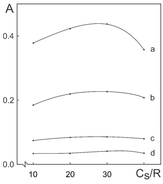
Figura 3 - Efeito da razão entre as taxas de fluxo C_S/R na resposta do sinal para 10,00 (a), 5,00 (b), 2,00 (c) e 1,00 (d) \mu\text{g/L} Hg.
